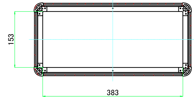
C-C ( 1 : 6 )
